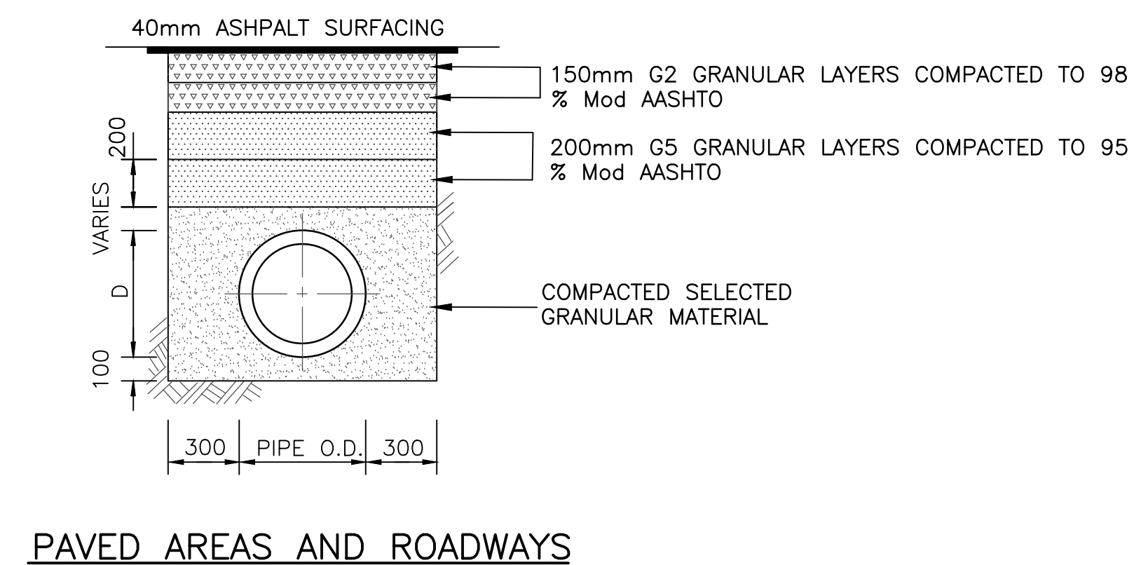
TYPICAL TRENCH SECTION N.T.S.
