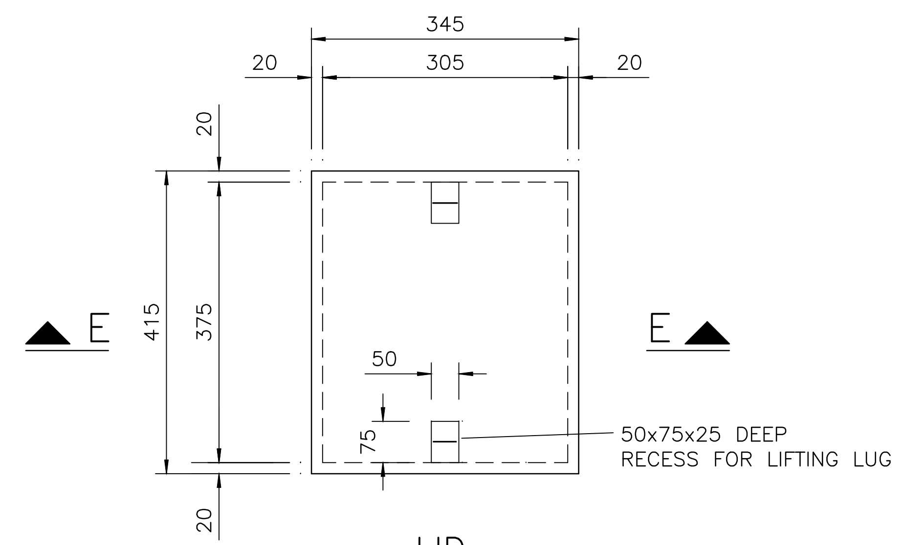
LID PLAN ON PRECAST LID 1 : 10
