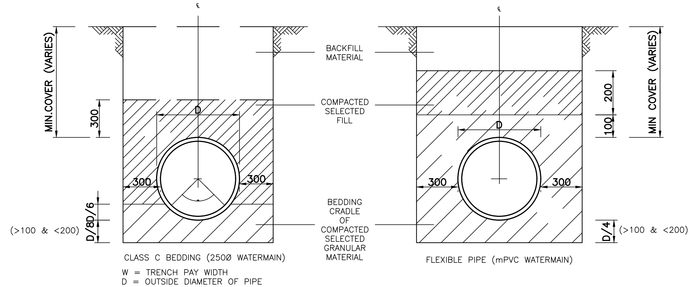
PIPE BEDDING DETAILS SCALE: 1:15
