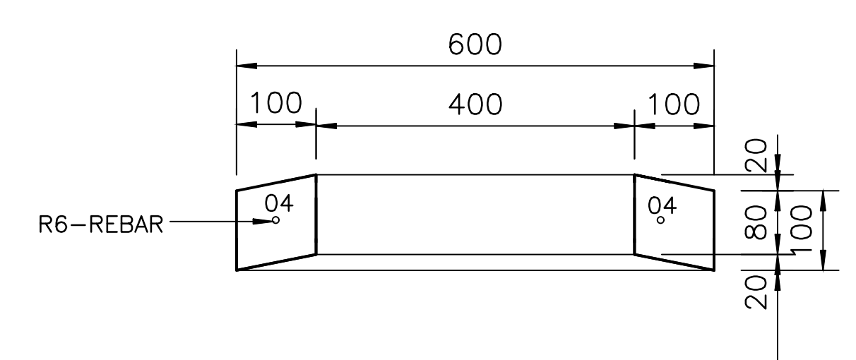
SECTION D-D 1 : 10
