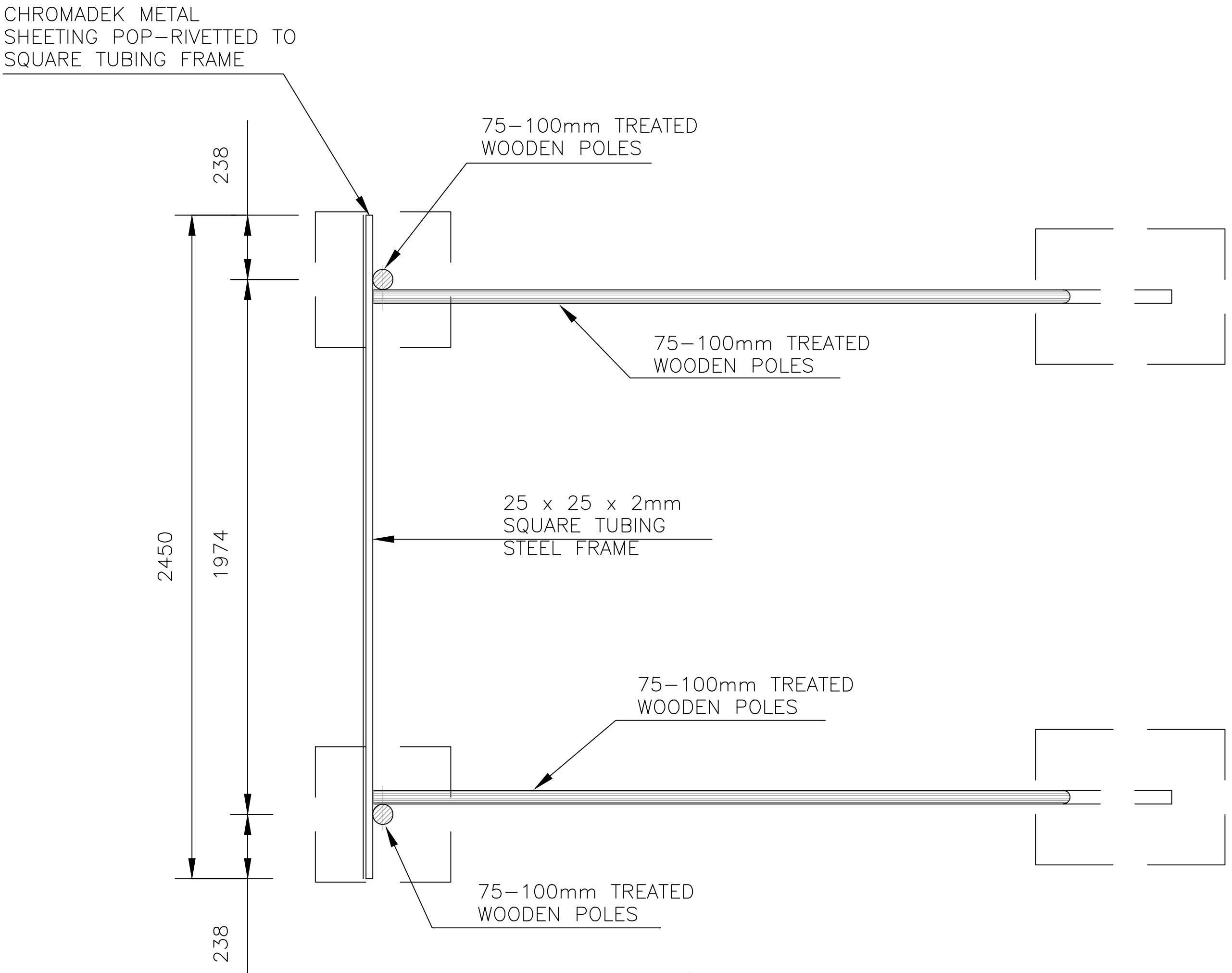
PLAN SCALE 1 : 20
