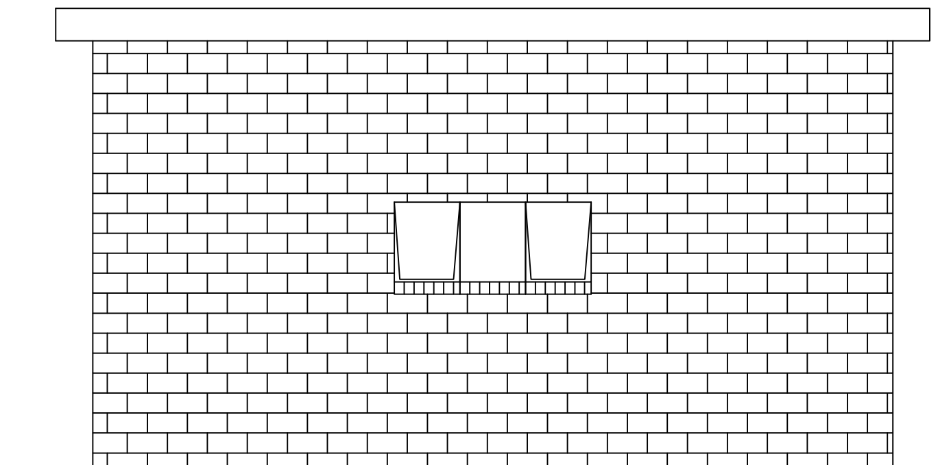
ELEVATION 1 1 : 50
